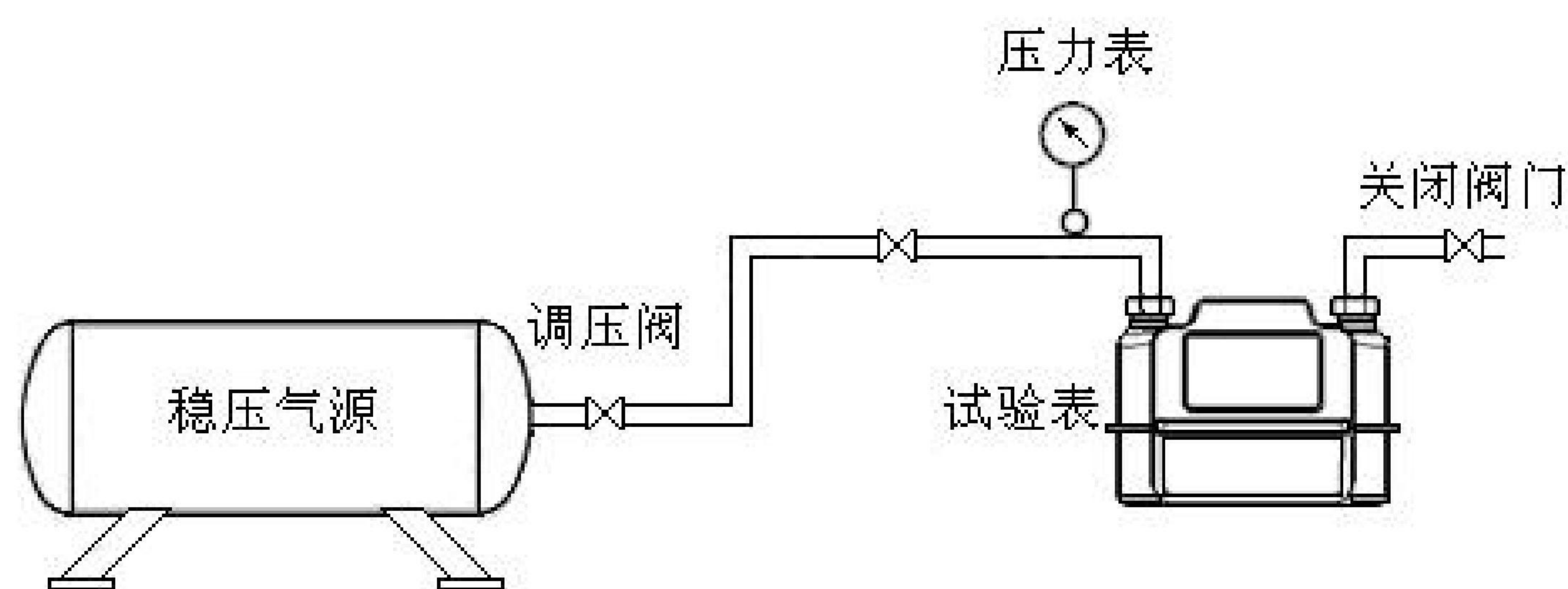
图 1 密封性试验示意图
