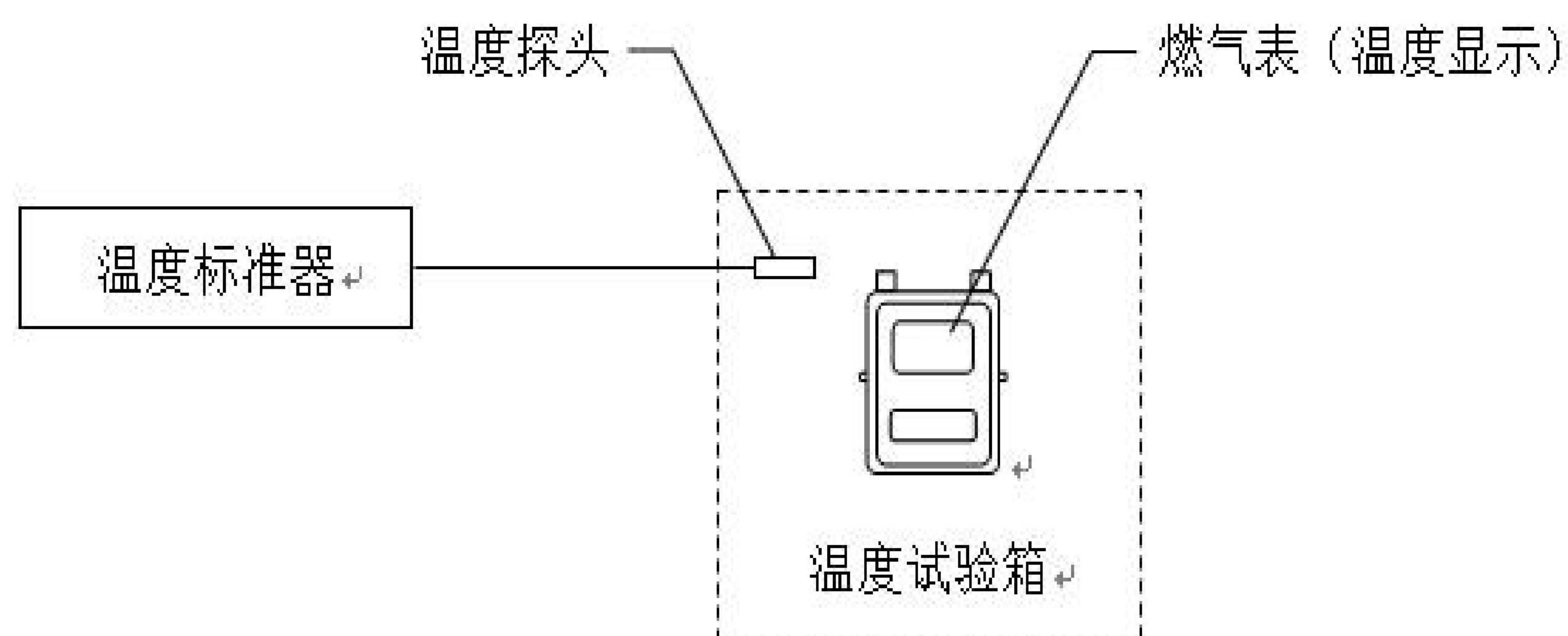
图 2 温度传感器检定示意图
