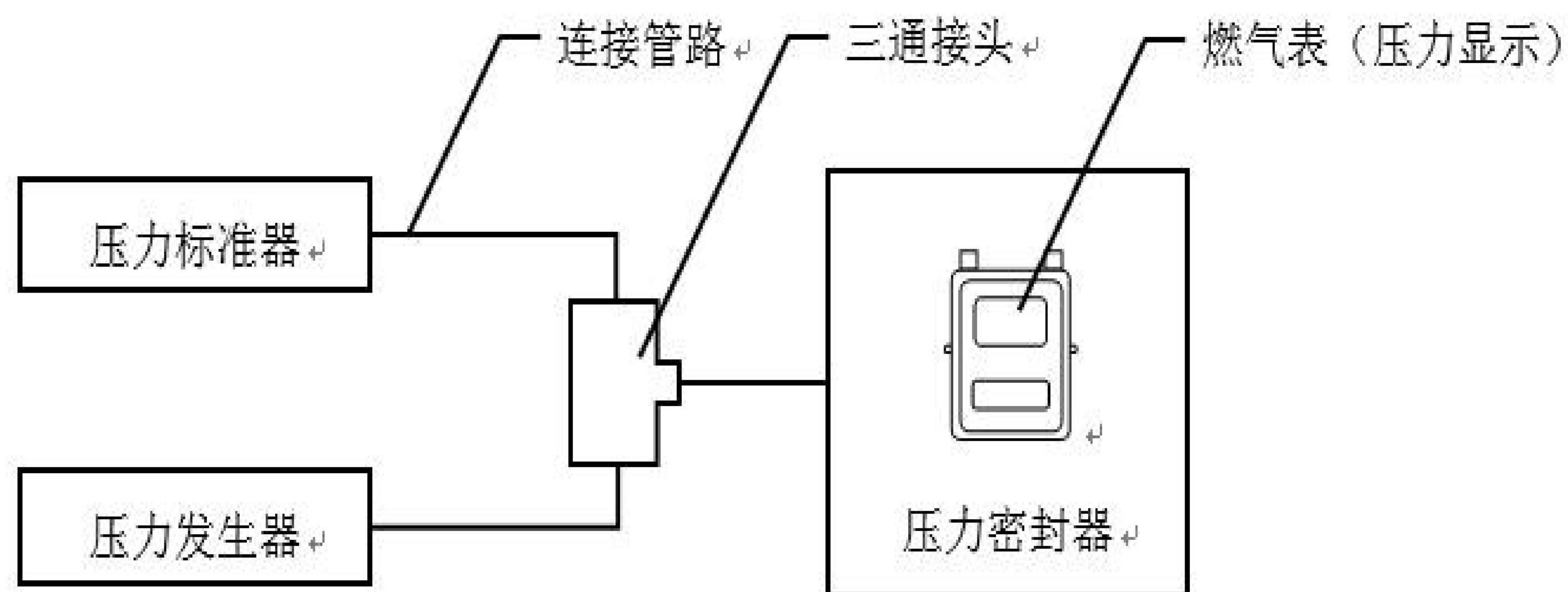
图 3 压力传感器检定示意图
